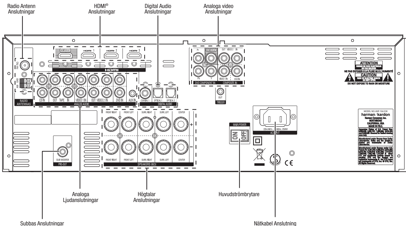
AVR 156 Baksidans Anslutningar
